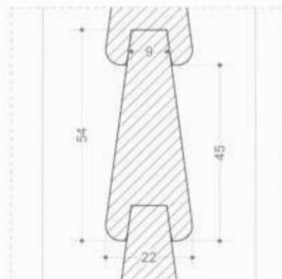
Particolare A
