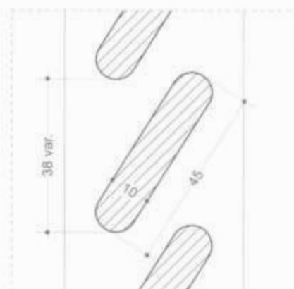
Particolare A
