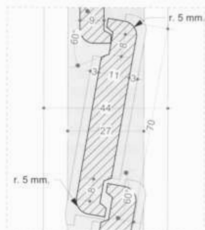
Particolare A
