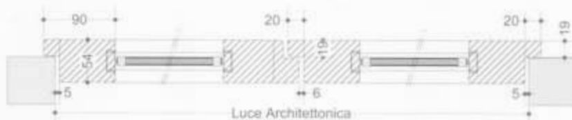
Sezione orizzontale
