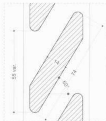
Particolare A
