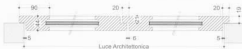
Sezione orizzontale
