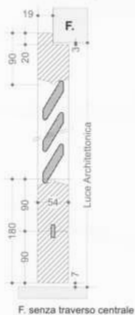
Sezione verticale
