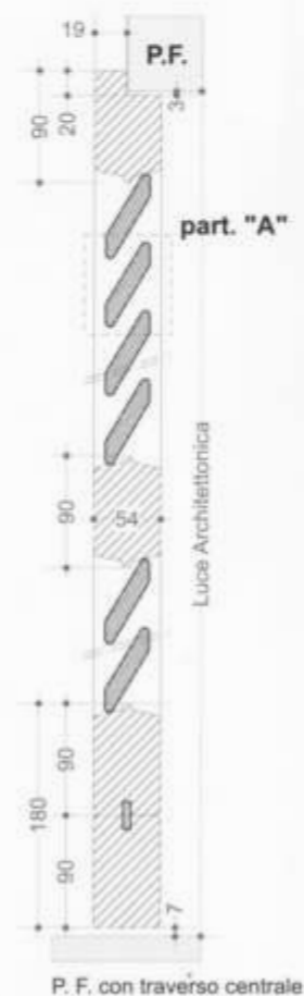
Sezione verticale
