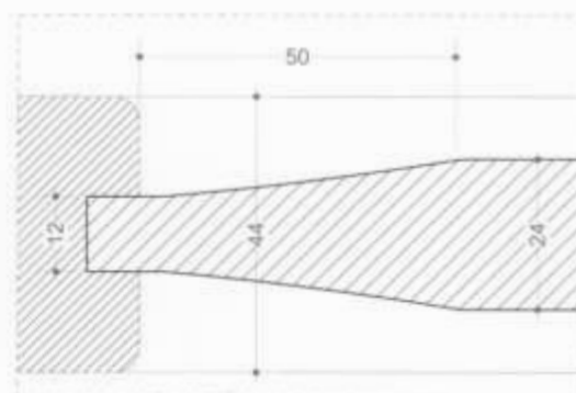
Particolare A
