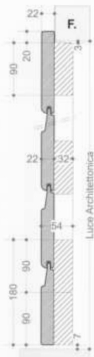
Sezione verticale
