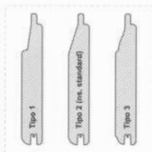
Sagome traversi
