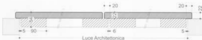
Sezione orizzontale
