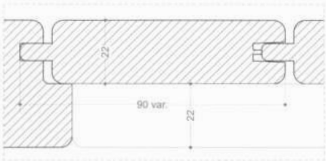
Particolare A
