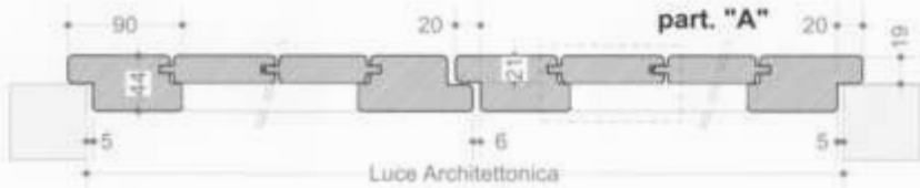
Sezione orizzontale
