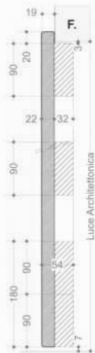
F. con traverso centrale
