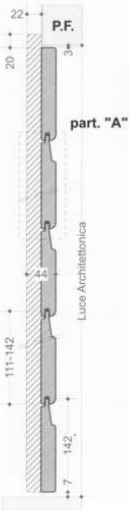
Sezione verticale
