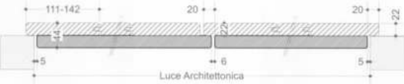
Sezione orizzontale
