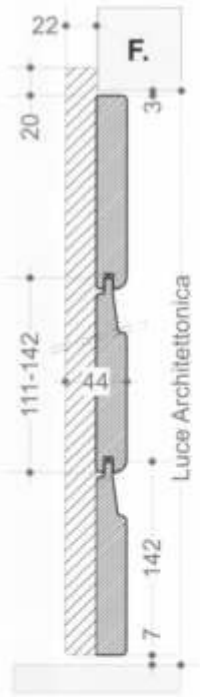
Sezione verticale
