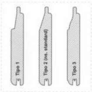
Sagome trasversi
