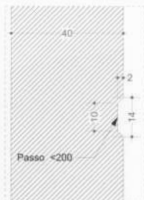
Particolare A
